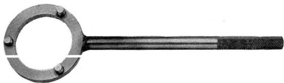
Levier à ergots pour maintenir le couvercle d'embrayage
